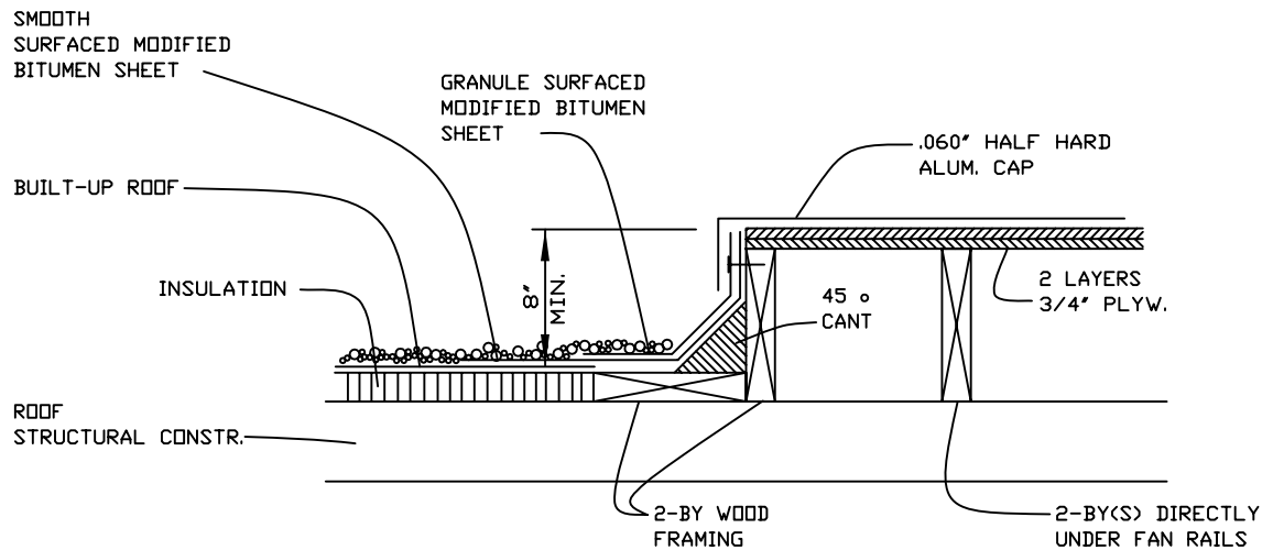
FAN CURB DETAIL
